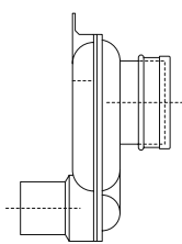
SIFONE PER ORINATOIO SIPHON KIT FOR URINAL IN DOTAZIONE / INCLUDED IN THE BOX
